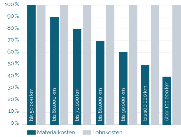
Materialkosten nach Betriebsleistung des beschädigten Bauteils
